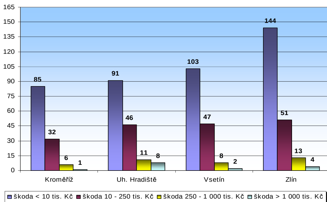
Graf 6 Srovnání počtu požárů podle přímé škody po okresech
