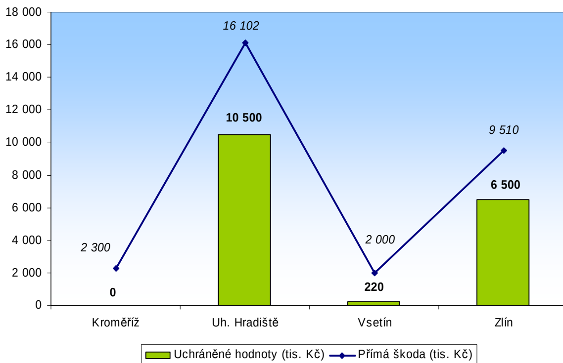
Graf 7 Přehled přímé škody a uchráněné hodnoty při požárech nad 1 mil. Kč po okresech
